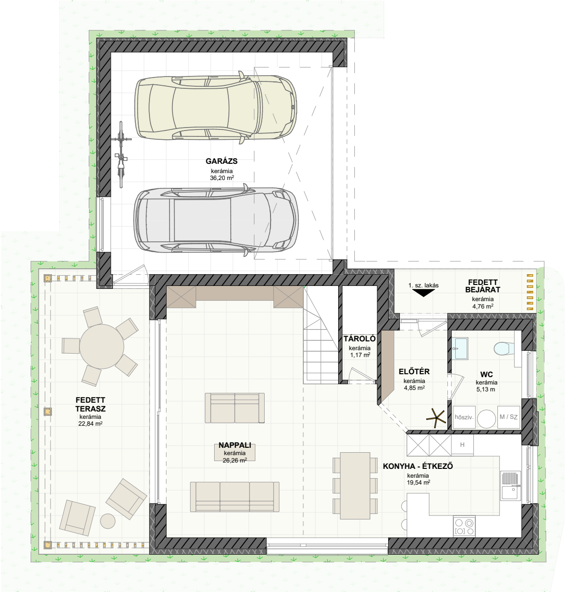
Földszinti alaprajz
