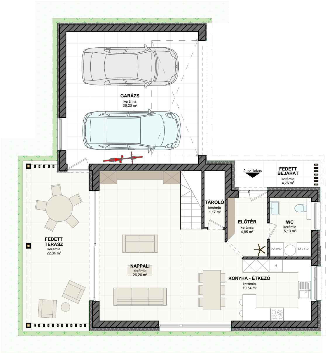
Földszinti alaprajz
