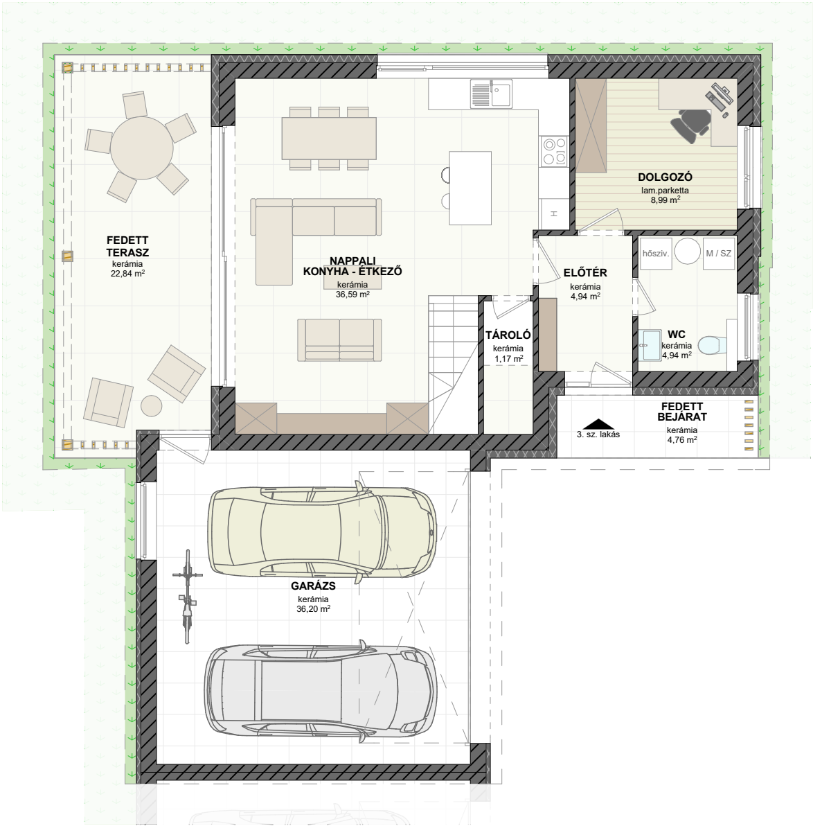
Földszinti alaprajz
