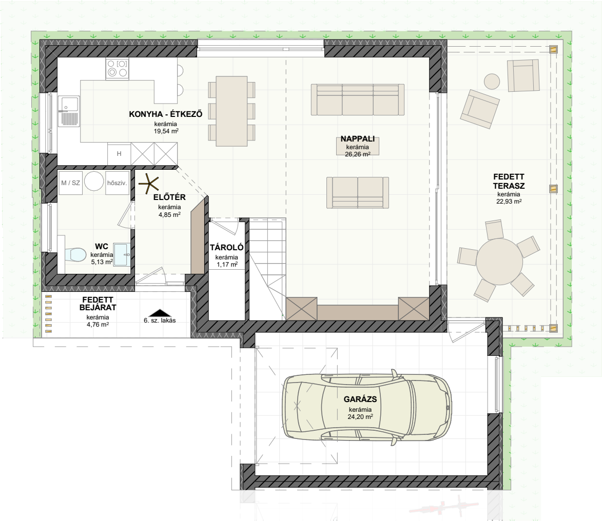
Földszinti alaprajz
